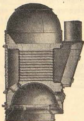
Cochrans pat. Donkey-Kjedel.
